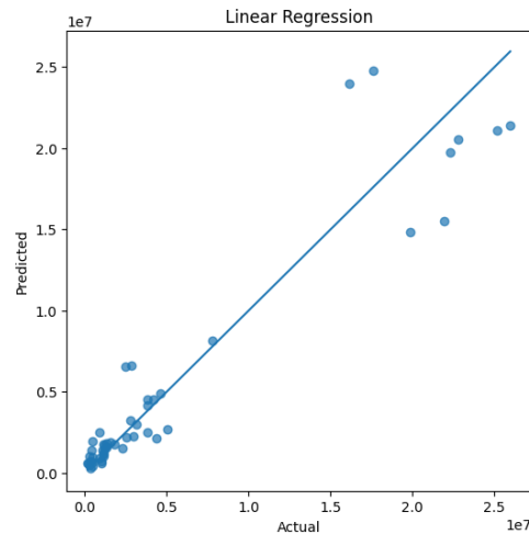
Gambar 3. Visualisasi Nilai Aktual dan Prediksi Linear Regression
